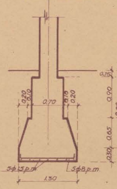
SECCIÓN III-III
