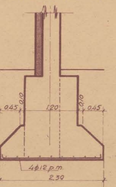
SECCIÓN II-II
