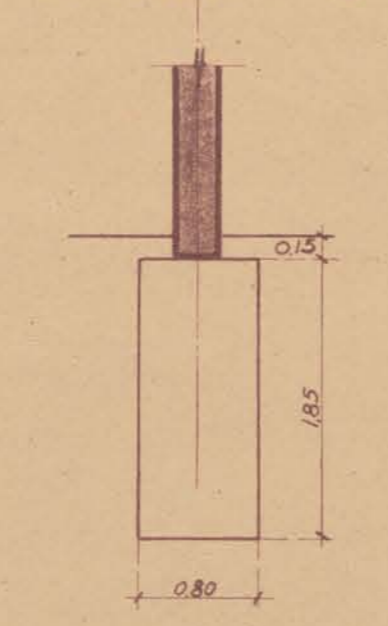
SECCIÓN V-V
