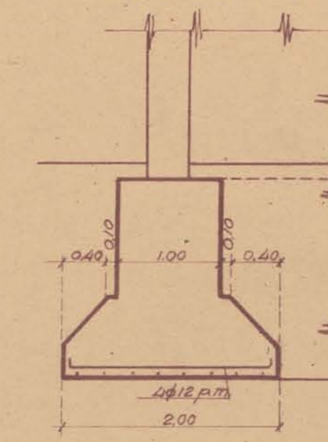
SECCIÓN I-I
